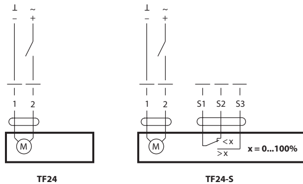
Схема электрических соединений
